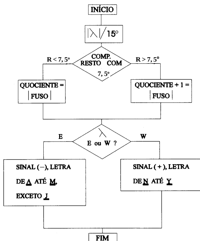
Figura 19.7 – Fluxograma para Determinação do Fuso Horário
